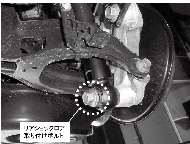
リアショックロア取り付けボルト 1カ所締め付け 締め付けトルク: 160N・m(16.3kgf・m)
