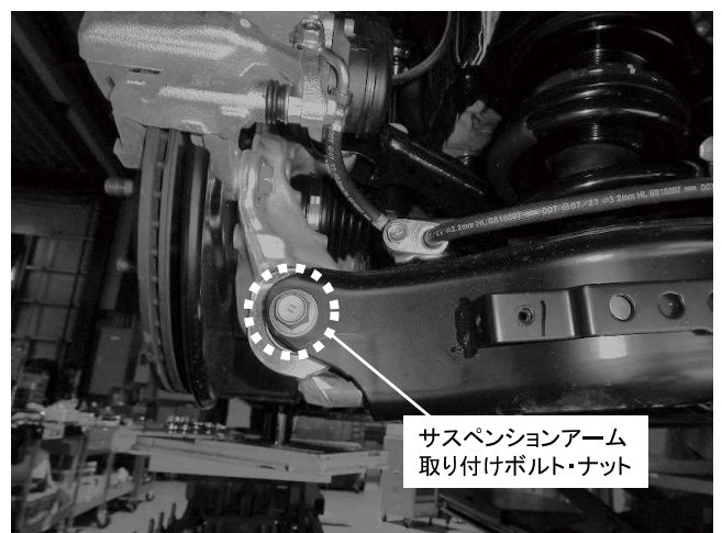
サスペンションアーム取り付けボルト・ナット 1カ所締め付け 締め付けトルク: 125N・m(12.7kgf・m)
