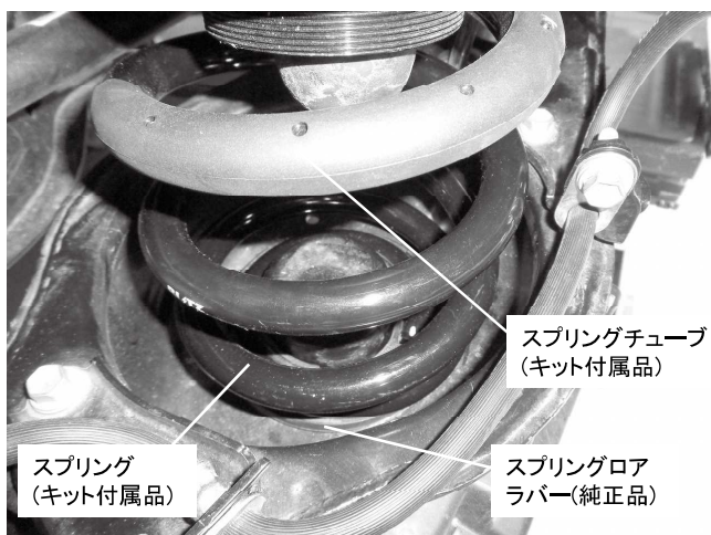
リアスプリングロー側取り付け状態 ※スプリングをサスペンションアームに取り付けの際 スプリング下部に純正スプリングローラバーを取り付けてください ※スプリングが線間密着する際、必要に応じてスプリング チューブを使用してください
