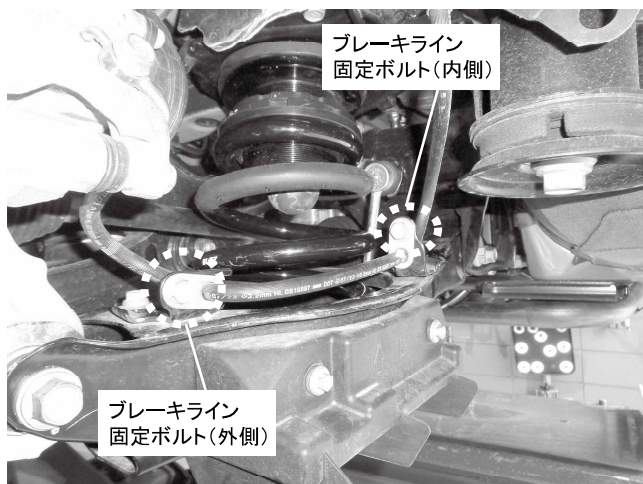
ブレーキライン固定ボルト 2カ所締め付け 内側締め付けトルク: 17.8N・m(1.8kgf・m) 外側締め付けトルク: 18.8N・m(1.9kgf・m) ※サスペンションアーム作業時必ず取り外してください 作業時にホースが引っ張られないよう注意してください
