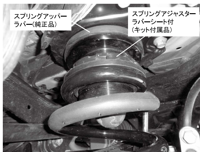
リアスプリングアッパー側取り付け状態 ※スプリングアジャスター取り付けの際アジャスター上部に 純正スプリングアッパーラバーを取り付けてください ※スプリング内純正バンブラバーはそのまま使用します
