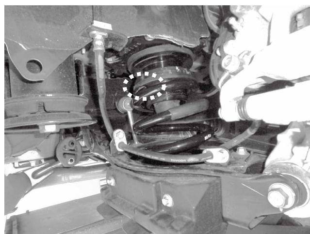
リアスプリング取り付け注意 ※リアスプリング取り付けの際アジャスターについている ラバーシートにスプリングが引っかかる可能性があります そのまま取り付けると異音の発生やラバーの破損に つながりますのでご注意願います
