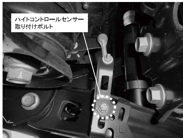
ハイトコントロールセンサー取り付けボルト(左側のみ) 1カ所締め付け 締め付けトルク: 12N・m(1.2kgf・m)
