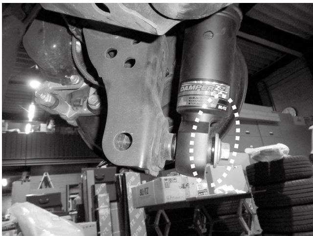
リアショック下側取り付け状態
