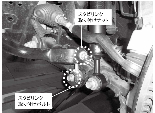
スタビリンク取り付けナット スタビリンク取り付けボルト スタビリンク取り付けナット 1カ所締め付け 締め付けトルク: 190N・m(19.4kgf・m) ※KDSS装着車 締め付けトルク: 128N・m(13.1kgf・m) ※KDSS未装着車 スタビリンク取り付けボルト 1カ所締め付け 締め付けトルク: 140N・m(14.3kgf・m)
