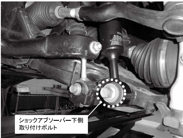
ショックアブソーバー下側 取り付けボルト ショックアブソーバー下側取り付けボルト 1カ所締め付け 締め付けトルク: 250N・m(25.5kgf・m)
