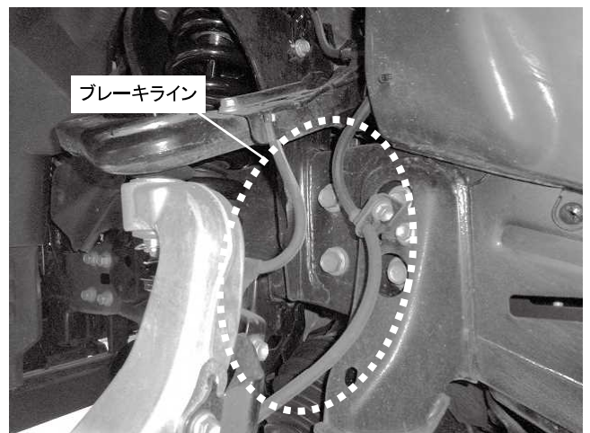
ブレーキライン フロントサスペンション脱着の際、 ブレーキラインやスピードセンサーの 破損に注意してください
