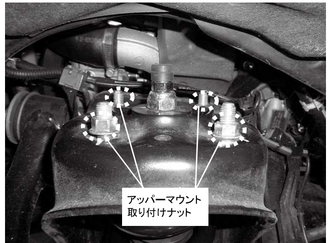
アッパーマウント取り付けナット 4カ所締め付け 締め付けトルク: 45N・m(4.6kgf・m) ※製品付属のM10ナットを使用してください ※4点の寸法は微妙に異なります 取り付けにご注意ください ※必ずキット付属のダイヤルカバーを取り付けてください ※確認車両データを確認して初めてご使用される際の推奨減衰力に合わせてください
