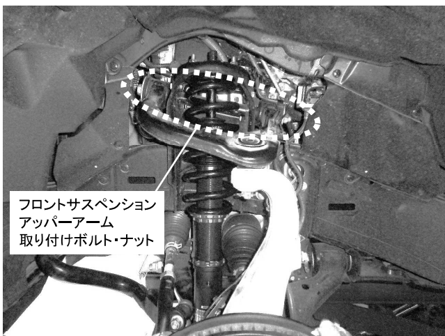
フロントサスペンション アッパーアーム 取り付けボルト・ナット フロントサスペンションアッパーアーム 取り付けボルト・ナット 1カ所締め付け 締め付けトルク: 185N・m(18.9kgf・m) ※ナット側を締め付けてください
