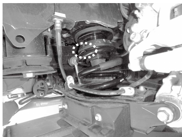
リアスプリング取り付け注意 ※リアスプリング取り付けの際アジャスターについている ラバーシートにスプリングが引っかかる可能性があります そのまま取り付けたら異音の発生やラバーの破損に つながりますのでご注意願います
