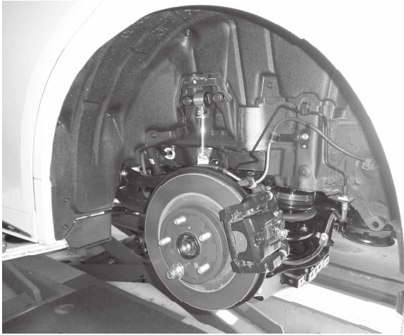
リア左側(助手席側)取り付け状態
